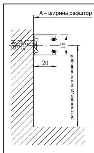
VL 1 — Направляющая для откосов
