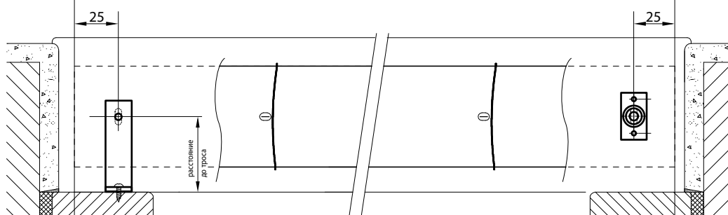
Установка тросовых направляющих, кронштейны троса DL и DL 4
