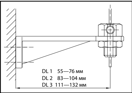
DL 1, DL 2, DL 3 — Кронштейн троса
