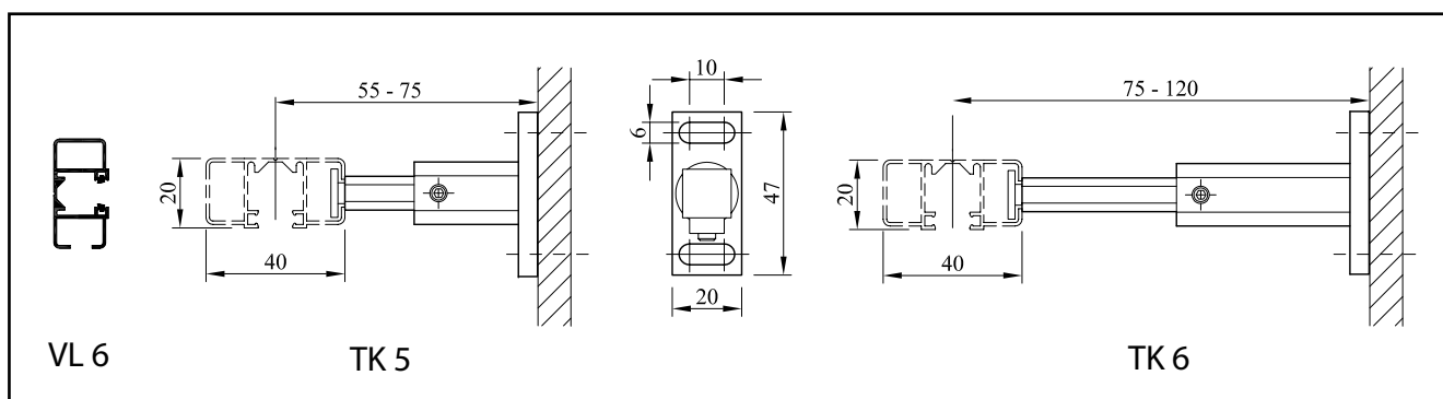
TK 5, TK 6 - раздвижной кронштейн для консольной направляющей VL 6
