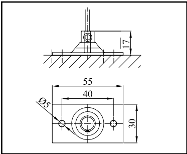
DL 4 — Кронштейн троса для крепления к полу
