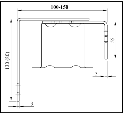
DK 5 — Раздвижной кронштейн короба
