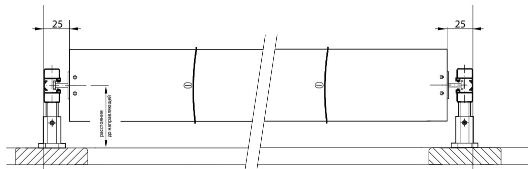
Установка направляющих VL 6 на оконную раму
