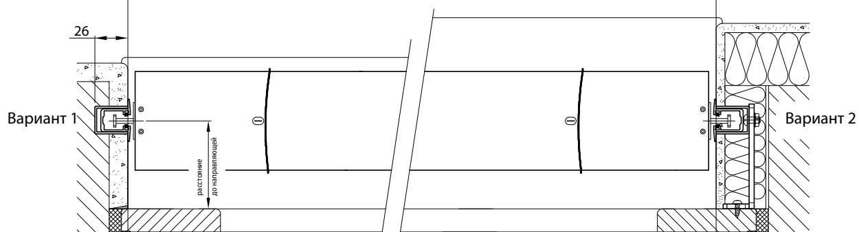
Установка направляющих VL 7 в откос / в откос с кронштейном К 4
