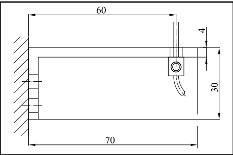
DL — Стандартный кронштейн троса
