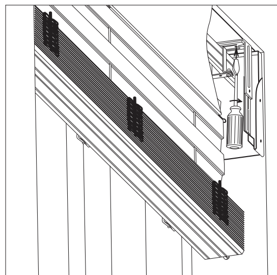
Закрепите защитный короб на кронштейнах.
