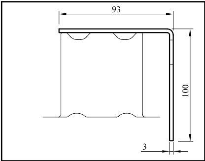
MD 2b — Настенный установочный кронштейн
