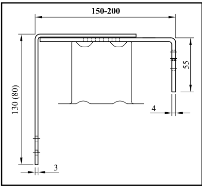
DK 6 — Раздвижной кронштейн короба
