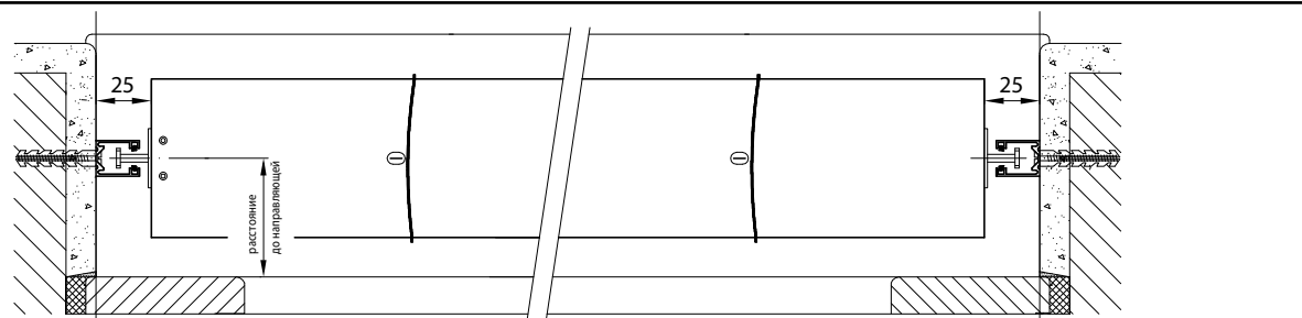
Установка направляющих VL 1 на откосы
