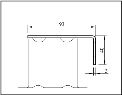
MD 2a — Установочный кронштейн для рамы
