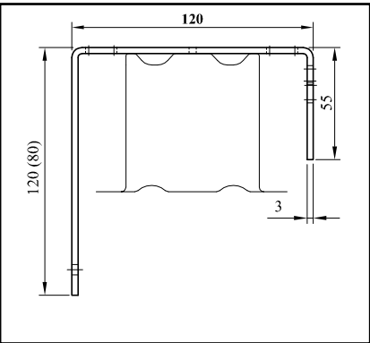
DK 3 — Кронштейн короба
