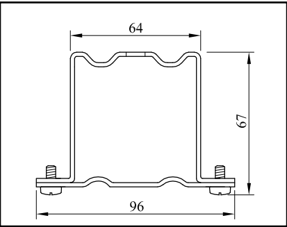
MD 1 — Стандартный установочный кронштейн
