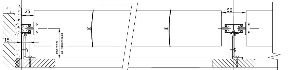
Установка направляющих VL 2 на кронштейны и направляющих VL 3 для соединения рафштор
